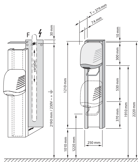
Douche à air chaud Vendaval réglable en hauteur, avec radar HF
