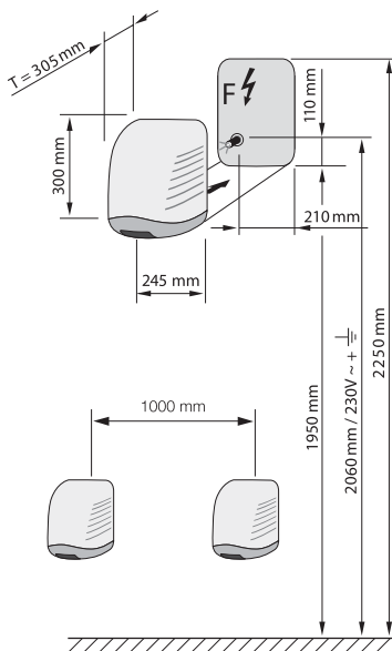
Douche à air chaud Vendaval, montage fixe, avec radar HF
